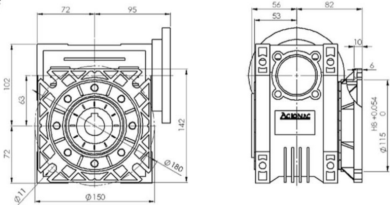
FCNDKO 63 F
